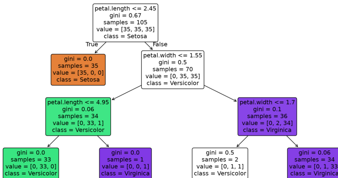
Рисунок 4 — Обученное дерево с ограничением глубины 3
