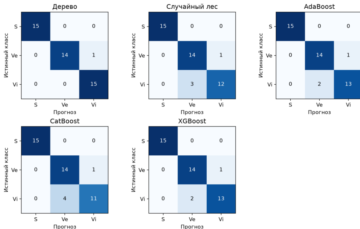
Рисунок 3 — Матрицы ошибок всех пяти классификаторов
