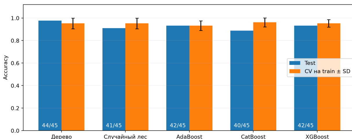
Рисунок 2 — Точность на тесте и при кросс-валидации train
